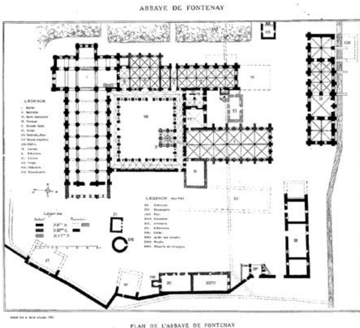
Grondplan van de abdij van Fontenay, opgesteld volgens de principes van Cîteaux. De gevangenis staat aangeduid met nummer XX onder de naam 'enfermerie'. (bron: L. Bégule, L'abbaye de Fontenay et l'architecture cistercienne (Lyon, 1912). Toegang via gallica.bnf.fr)
